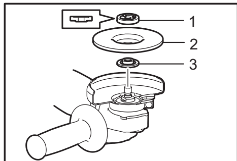
► 1. Contratuercas 2. Disco de centro hundido 3. Brida interior
