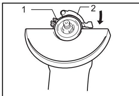
► 1. Screw 2. Lever
