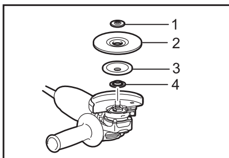
► 1. Contratuercas 2. Disco flexible 3. Almohadilla de soporte 4. Brida interior
